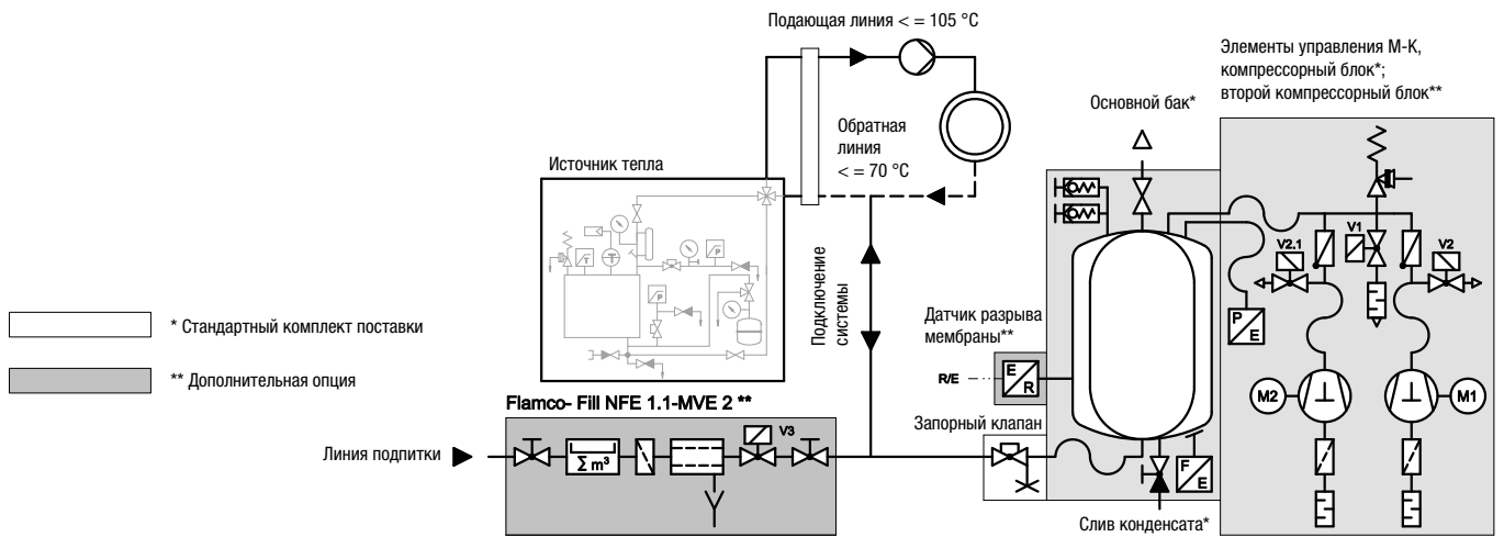
Принципиальная схема подключения АУПД Flexcon M-K/U с двойным компрессорным блоком и основным баком для системы отопления с отдельным блоком подпитки
