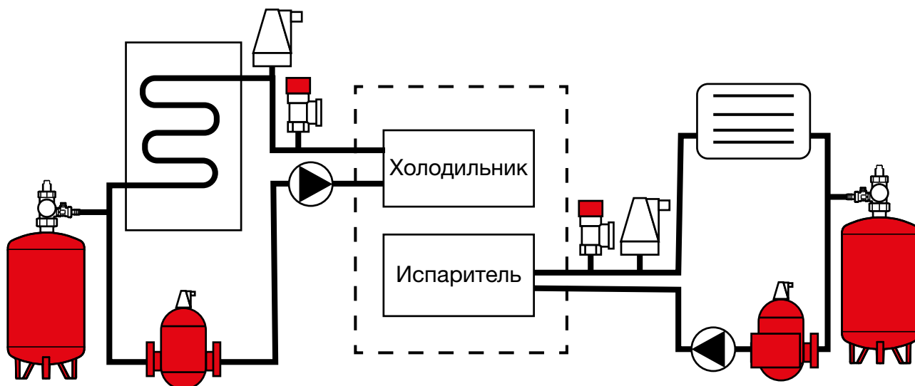
Система холодоснабжения
